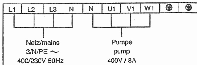
Anschluss einer 400V Drehstrompumpe
