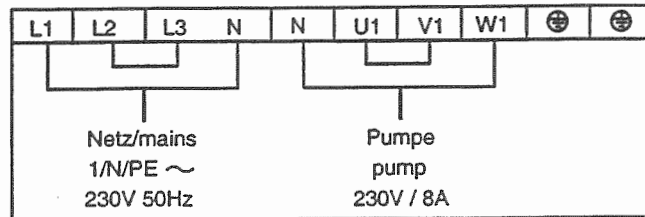
Anschluss einer 230V Wechselstrompumpe
