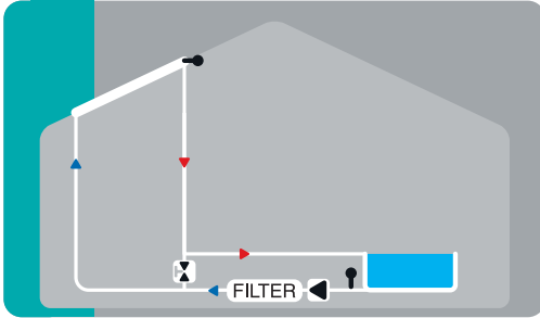
Pool+Solar / Solar mit Ventil und Filterpumpe und Pool
