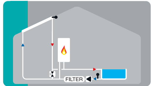
Pool + Solar + Zusatzheizung / Solar + Zusatzheizung mit Ventil und Filterpumpe und Pool
